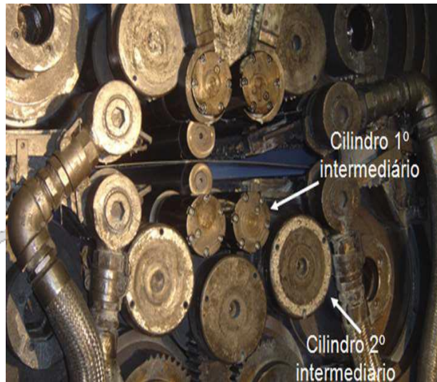
Cadeira do Sendzimir 2 aberta e no detalhe os cilindros 1º e 2º Intermediários em utilização. Podemos ver a chapa de aço em seu interior.
