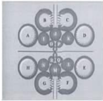
Esquema de posição dos cilindros em uma cadeia de Laminador.
